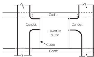
VUE LATÉRALE (VERS L'ARRIÈRE DU VR)
