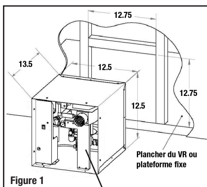
Ferrure de soutien/tuyau d'échappement de la soufflerie
